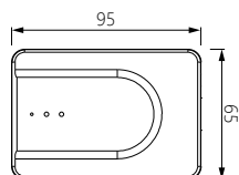
网关产品尺寸
